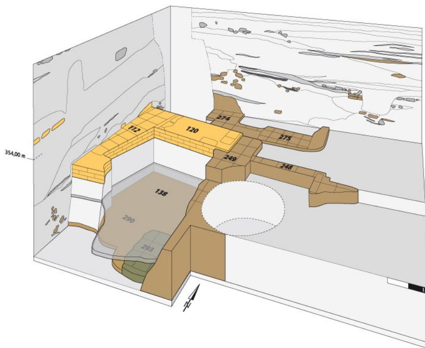
شكل ثلاثي الأبعاد للقطاع (B) (by artefacts-berlin). Fig. 4:
